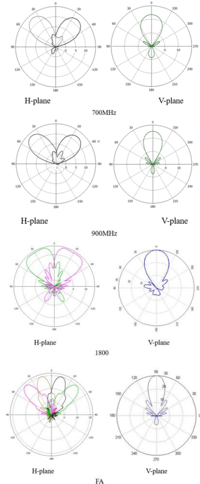
天线方向图示意图 Patterns
