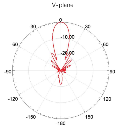
天线方向图示意图 Patterns
